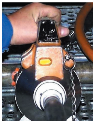
Figure 5 – Signal jaune : le projecteur est sur le chantier, la source rentrée et l'appareil déverrouillé par sa clé de sécurité individuelle. Yellow signal: the camera in on work place, source inside, and un-locked.
